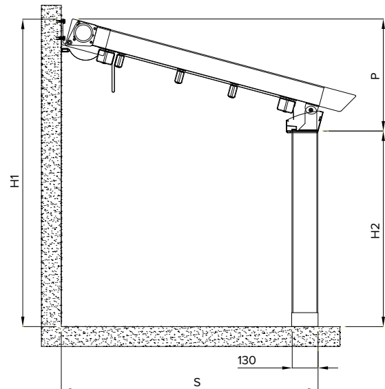
Vista laterale . Seitenansicht
