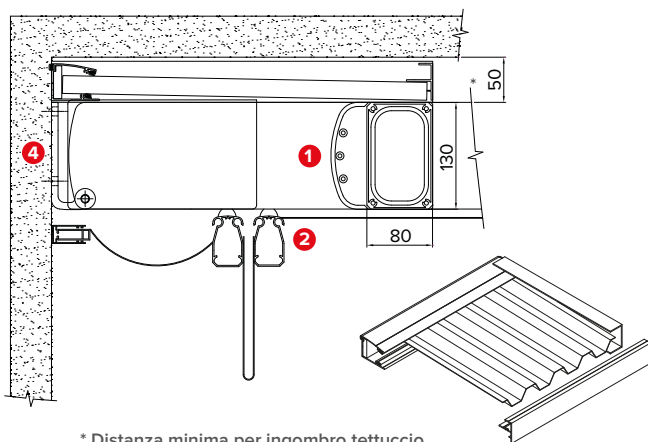
Dettaglio tettuccio . Detailansicht des Schutzdaches 033-977 / 033-978
