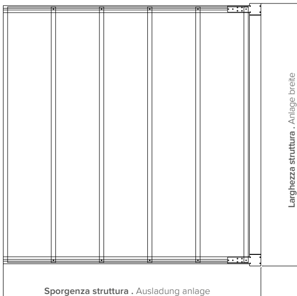
Vista dall'alto . Draufsicht
