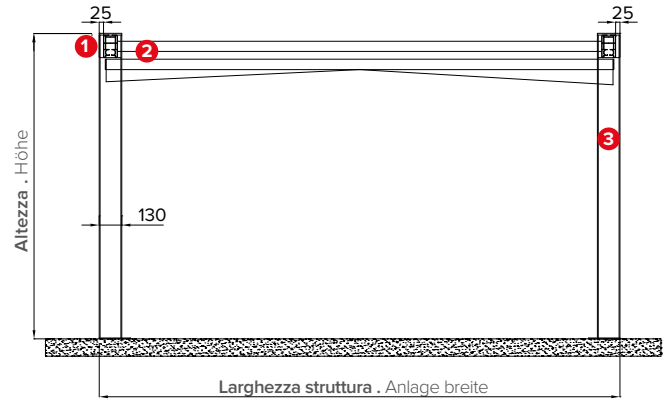
Vista frontale . Vorderansicht
