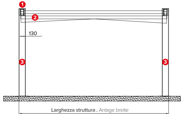
Vista frontale . Vorderansicht
