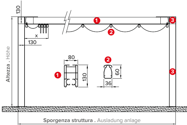
Vista laterale . Seitenansicht
