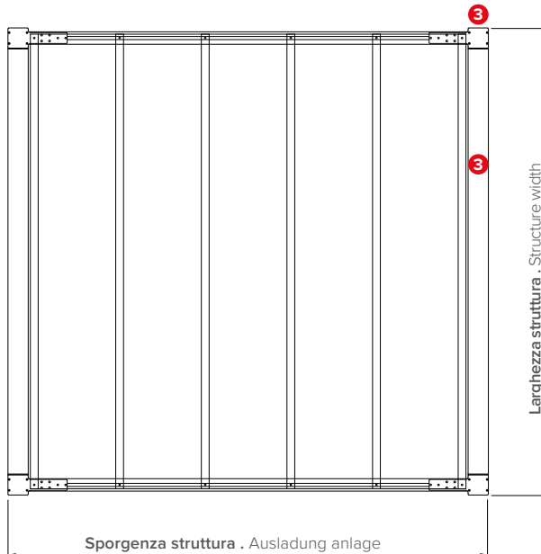
Vista dall'alto . Draufsicht
