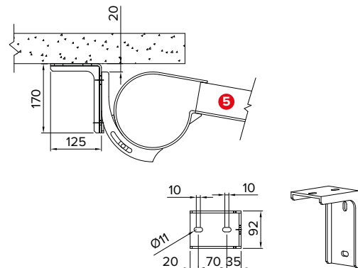
Attacco a soffitto . Deckenbefestigung 088-920
