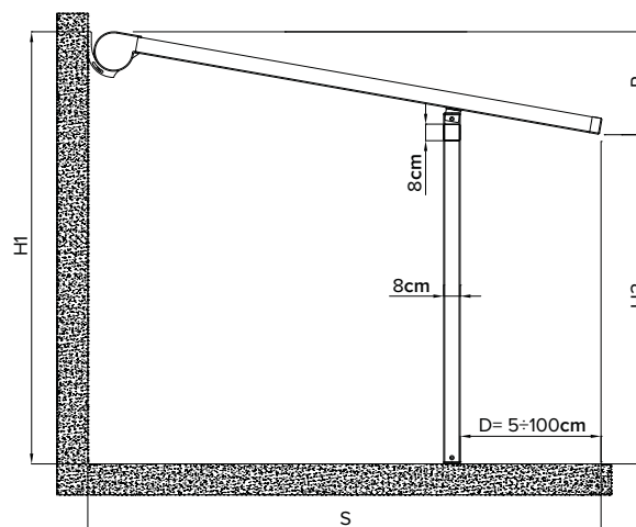
Vista laterale . Seitenansicht
