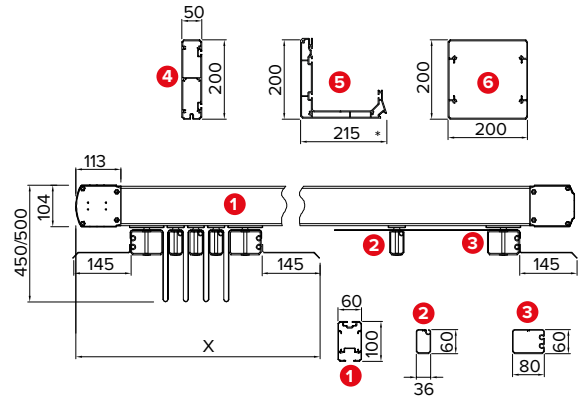
Dettaglio tettuccio . Detailansicht des Schutzdaches 033-986 / 033-987 / 033-988
