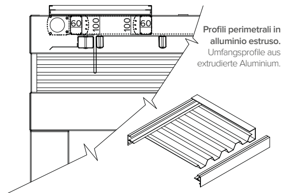
Dettaglio tettuccio . Detailansicht des Schutzdaches 033-986 / 033-987 / 033-988
