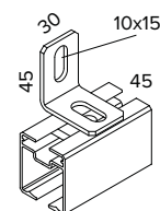
Attacco spallina Befestigung zwischen zwei Wänden
