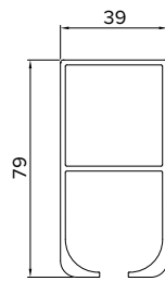
Guide Laterali Seitliche Führungen
