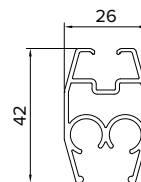
Profilo a 2 ogive Profil mit 2 Nuten
